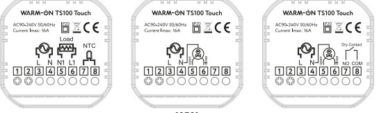
WE elektrische Heizung WW Wasserheizung WW-LD Heizkessel und Wasserheizung
