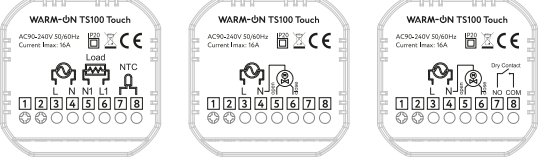
WE Chauffage électrique WW Chauffage à eau WW-LD chauffage de chaudière et chauffage à eau
